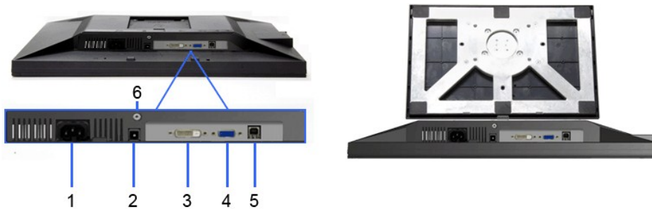
Tampilan Bawah
